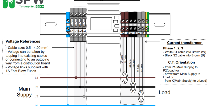
Wiring Diagram MKDVO45
