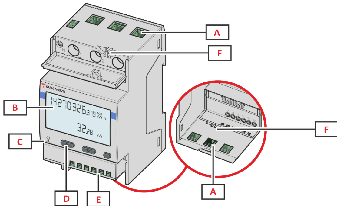
Abbildung 2 EM540 – Vorderseite
