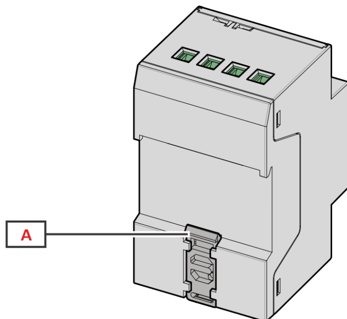
Abbildung 3 EM530/EM540 – Rückseite
